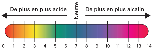
Échelle de pH
